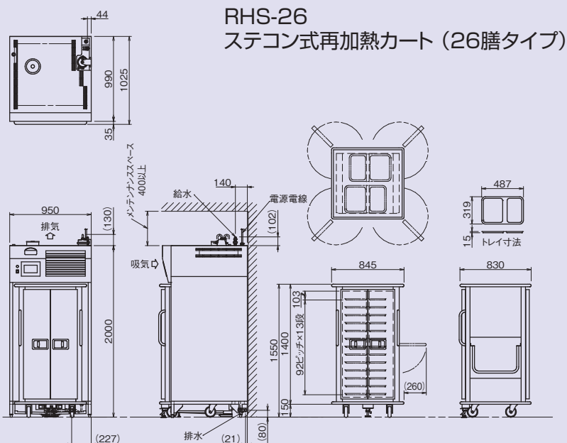
RHS-26 カート
